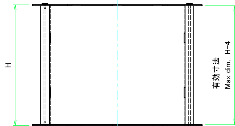
Wパネル1 / W panel 1
