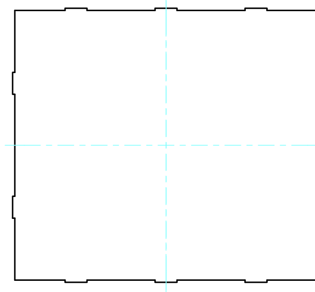
Dパネル2表面 / D panel 2 Frontside
